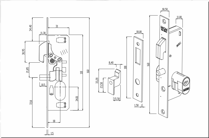
FECHADURA BICO DE PAPAGAIO
