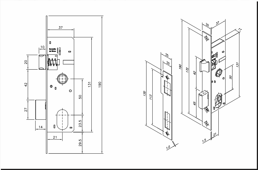
FECHADURA BROCA 40MM
