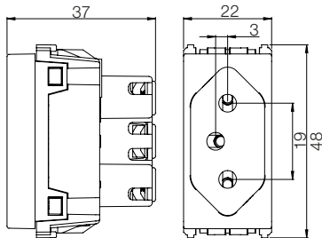
Tomada 2P+T-10 A
