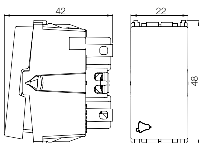
Pulsador Campainha (com ou sem LED)
