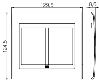
Placa 4x4 - 6 Posições
