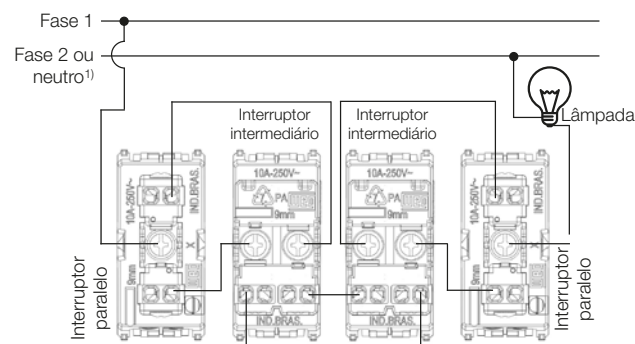
Dois Intermediários e Dois Paralelos
