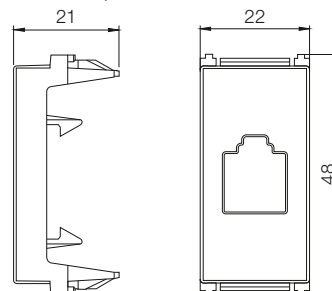
Módulo para RJ45
