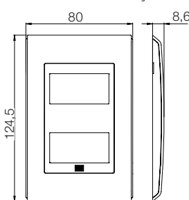
Placa 4x4 - 6 Posições
