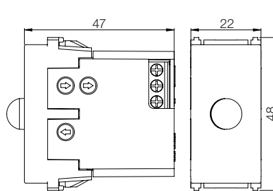
Sensor de Presença
