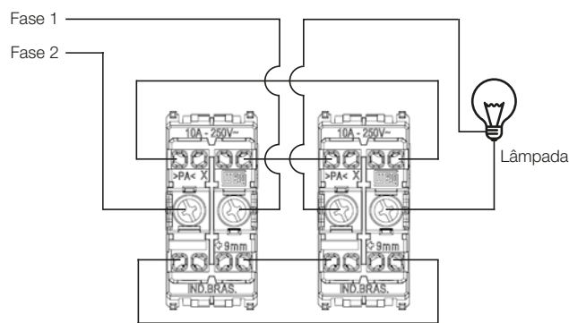
Interruptor Bipolar Paralelo
