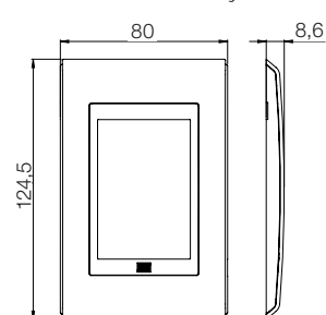
Placa 4x2 - 3 Posições
