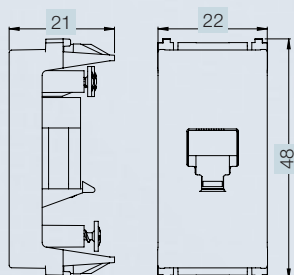
Módulo RJ11
