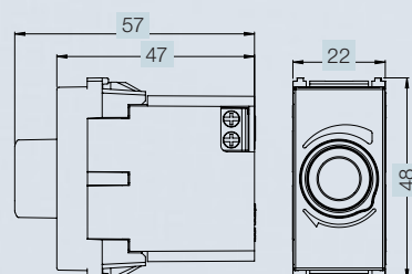
Módulo Dimmer
