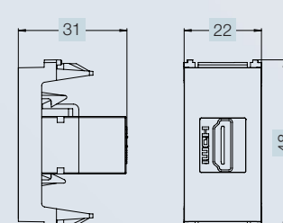
Módulo HDMI
