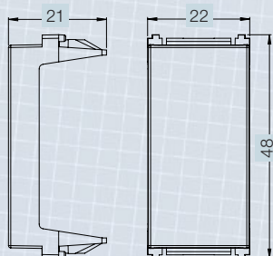
Módulo Cego
