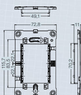
Suporte 4x2
