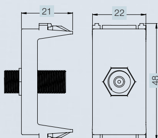
Módulo Antena
