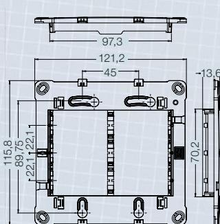
Suporte 4x4
